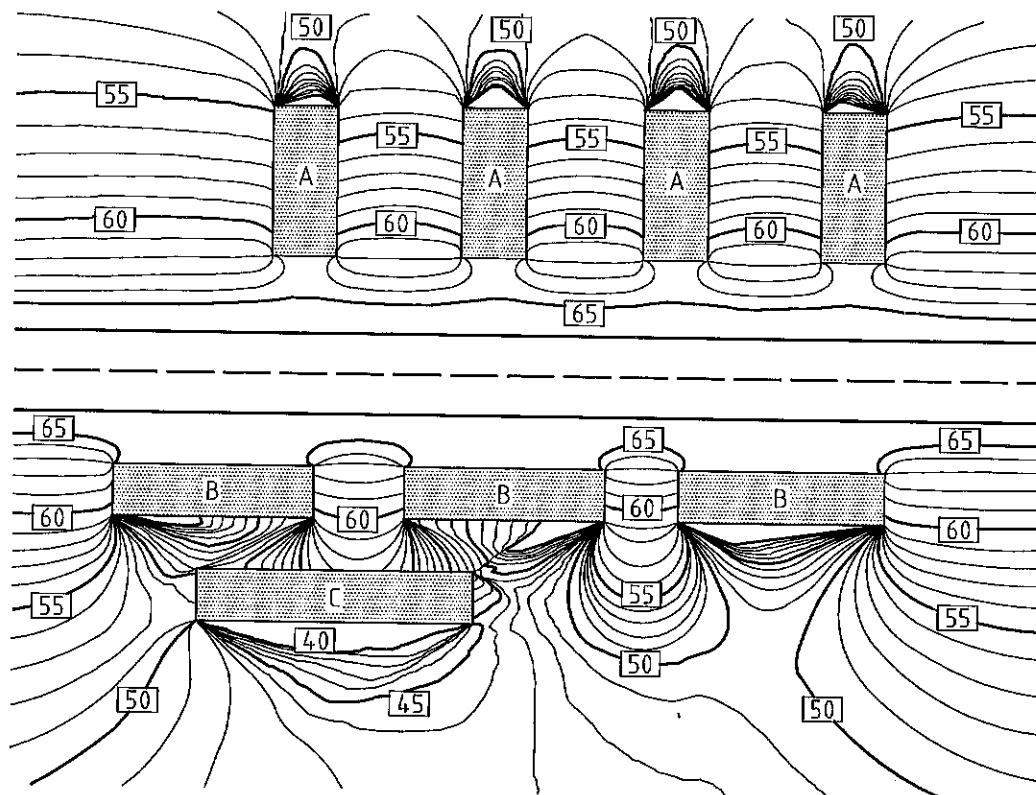
Bild 8 – Einfluss der Anordnung von Gebäuden auf die Schallausbreitung
