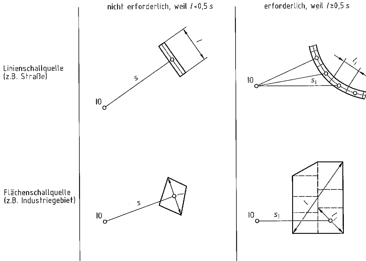
Bild 2 – Unterteilung in Teilschallquellen
