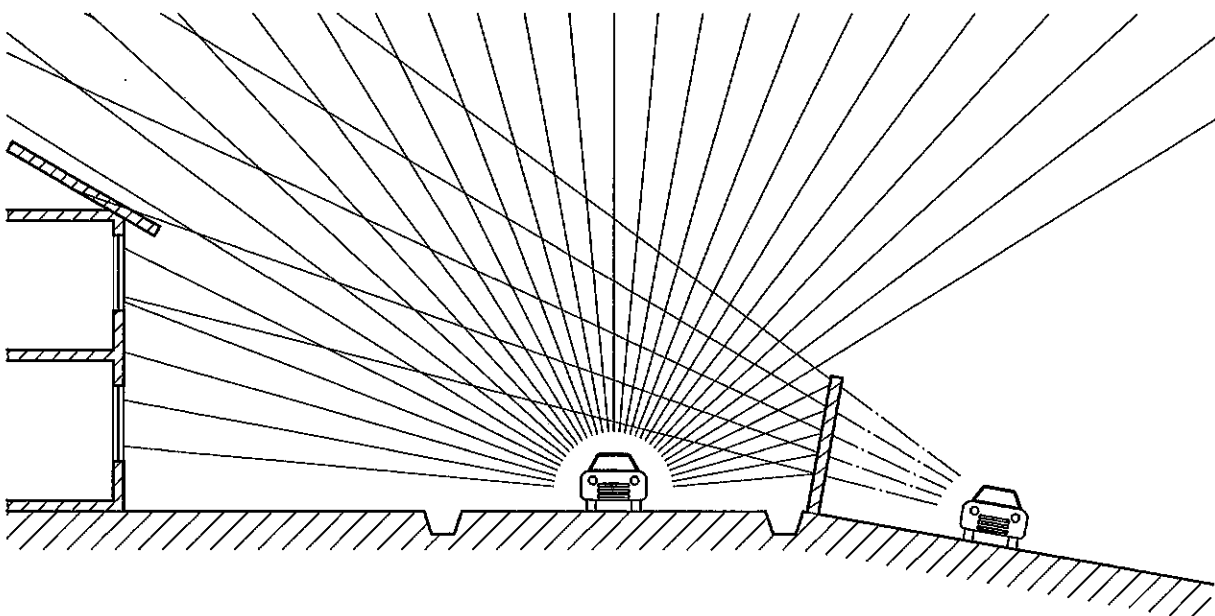
Bild 7 – Neigung einer Schallschutzwand
