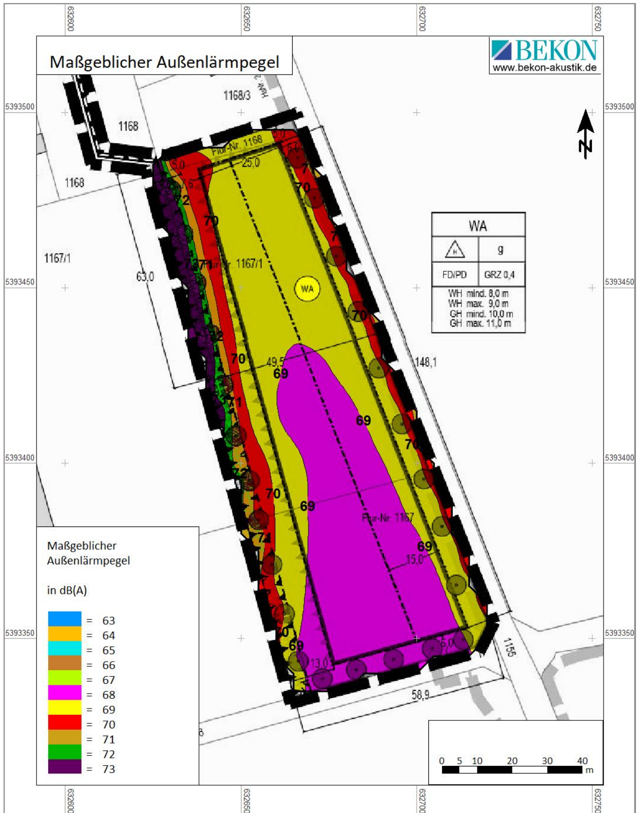
Abbildung 1: Maßgebliche Außenlärmpegel
