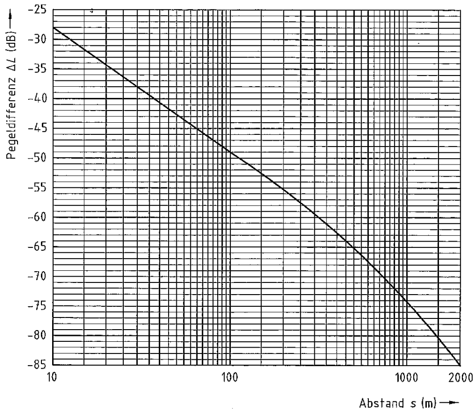
Bild 1 – Differenz \Delta L zwischen dem von einer Punktschallquelle am Boden bei ungehinderter Schallausbreitung ohne Zusatzdämpfung durch Boden- und Wittereinflüsse erzeugten Beurteilungspegel und ihrem Schalleistungspegel als Funktion des Abstandes s ( \Delta L = - [10 \lg(2 \cdot \pi \cdot s^2 / 1 \text{ m}^2) + s/200 \text{ m}] dB gilt für Verkehrs- und Anlagengeräusche)
